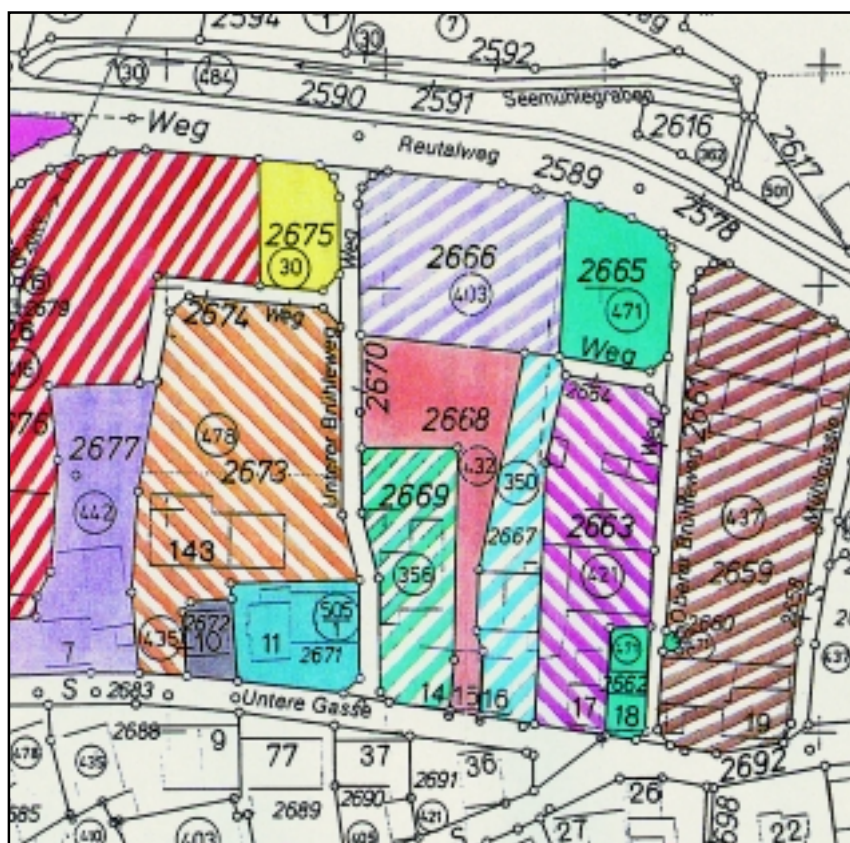
Oberstetten nach der Flurneuordnung
